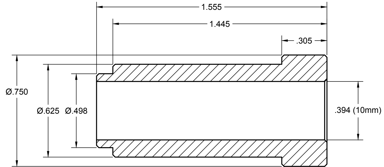
SECTION A-A SCALE 3:1
